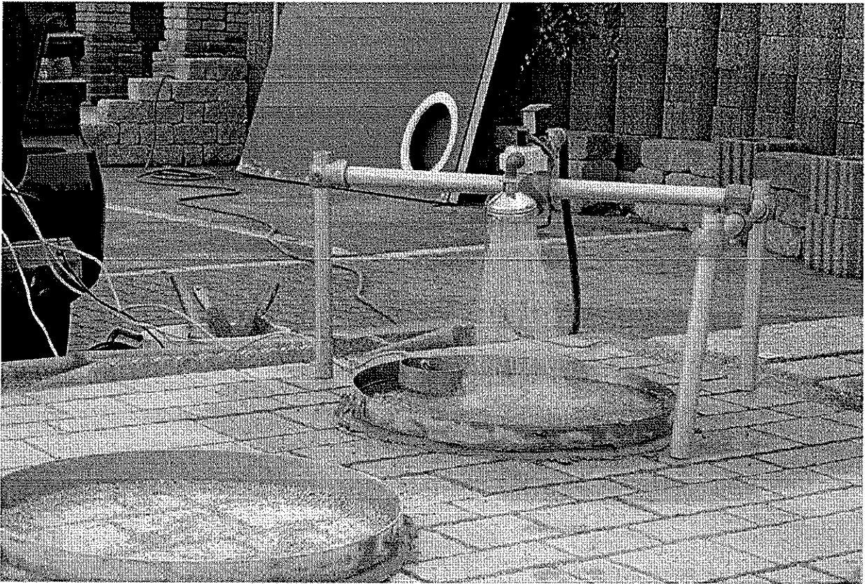
Bild 3: Untersuchungsgerät
