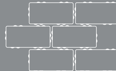
Rechteckpflaster mit Verschiebesicherung Verlegung im Kreuzfugenverband
